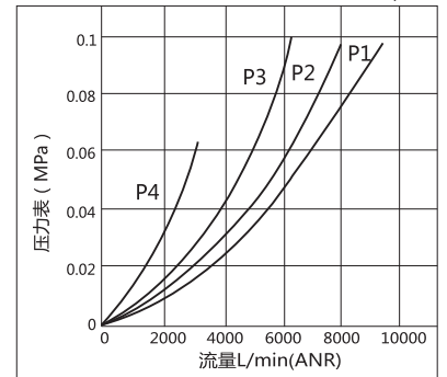
AF5000 3/4-1
